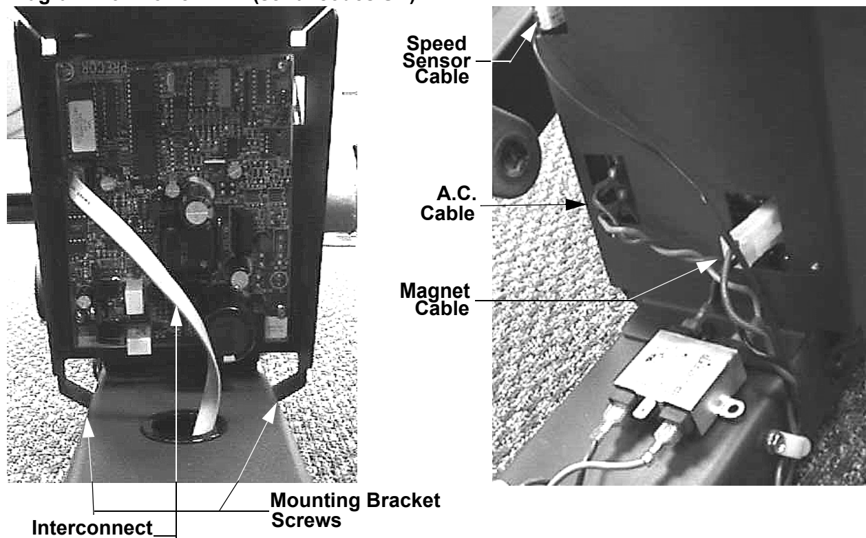
Diagram 7.3 - Lower PCA (serial codes SB)
